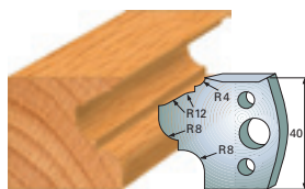
Coltelli Limitatori SN 089 K SO 089 K
