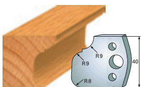
Coltelli Limitatori SN 068 K SO 068 K
