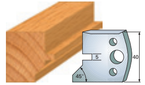
Coltelli Limitatori SN 083 K SO 083 K
