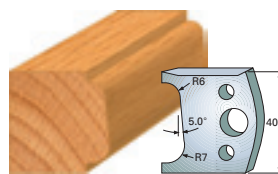
Coltelli Limitatori
