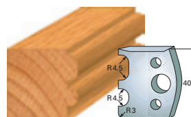
Coltelli Limitatori
