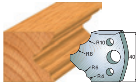
Coltelli Limitatori SN 125 K SO 125 K
