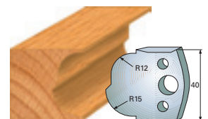
Coltelli Limitatori SN 115 K SO 115 K
