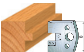
Coltelli Limitatori SN 092 K SO 092 K
