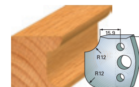
Coltelli Limitatori SN 176 K SO 176 K
