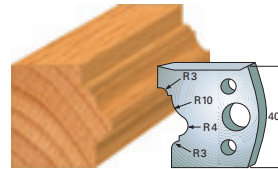
Coltelli Limitatori SN 102 K SO 102 K
